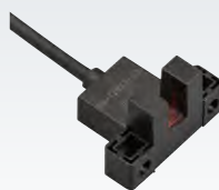
C3-SX671 槽型光电开关 尺寸：18.7×26.2×15.5mm
