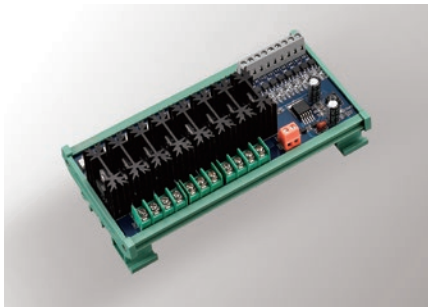
HHN-SL3 PLC 直流大功率放大板
