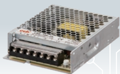
LRS-100W 单组输出超薄开关电源
