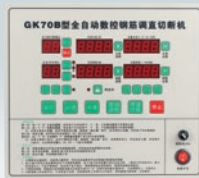
GK70B/GK70C 全自动数控钢筋调直切断机控制器 GK70B 带油泵电机和主机 GK70C 带主机
