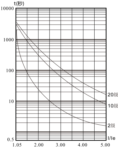
电机热保护脱扣时间曲线(热状态)
