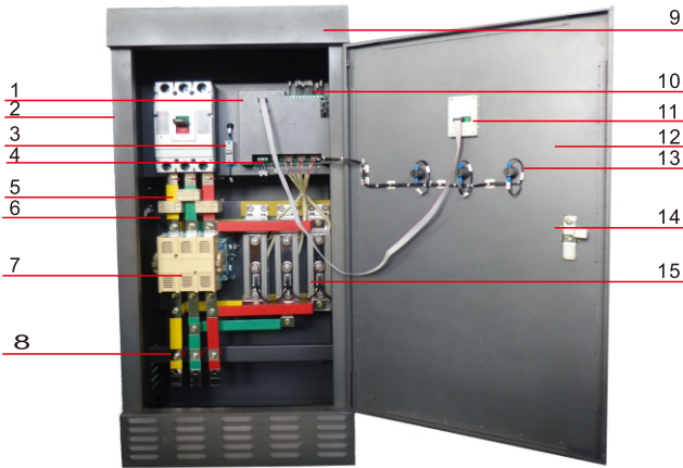
图1 机器外观图
